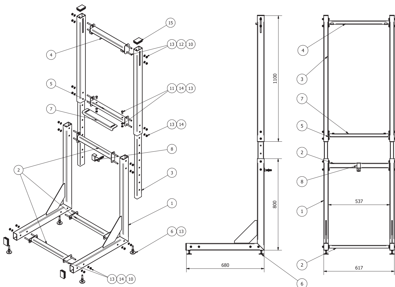
Rysunek złożeniowy stojaka dla kotła Victrix Pro 100-150
