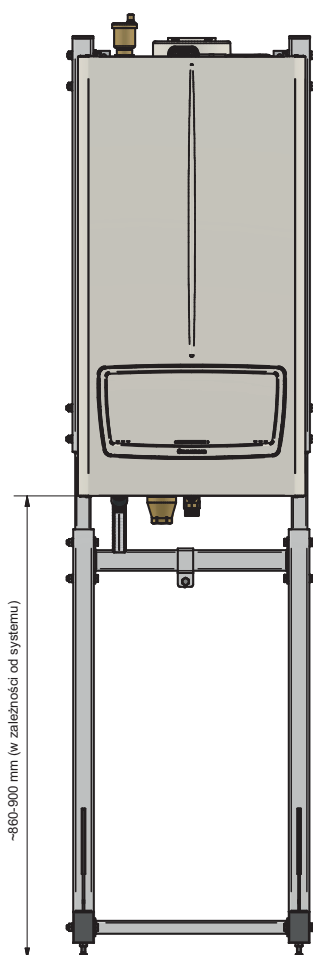
montaż z łącznikami S
