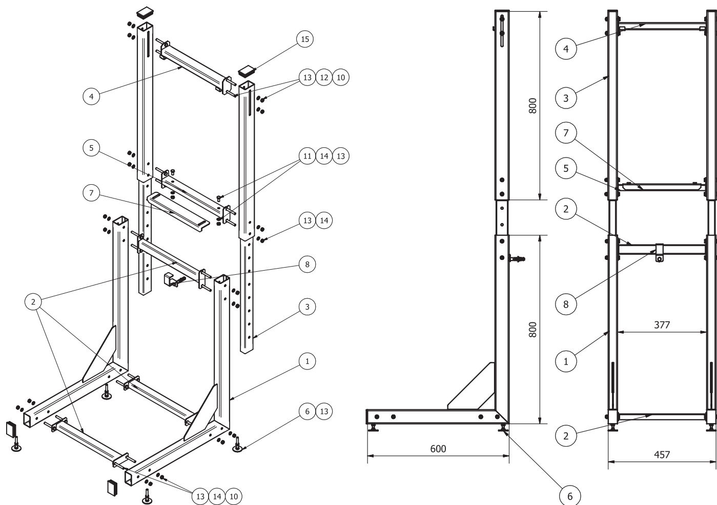
Rysunek złożeniowy stojaka dla kotła Victrix Pro 35-80
