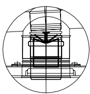
Szczegół "A" Klapa odcinająca
