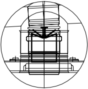
Szczegół "A" Kłapa odcinająca
