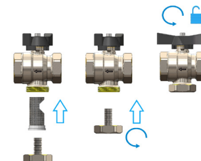
Rys. 9. Schemat złożenia zaworu kulowego BFV
