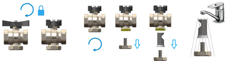
Rys. 7. Schemat konserwacji zaworu kulowego BFV
