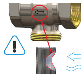
Rys. 8. Poprawne ułożenie filtra siatkowego
