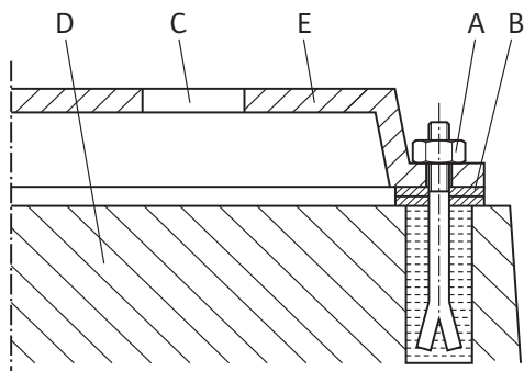
Fig. 8: Przykład połączenia śrubowego z fundamentem
