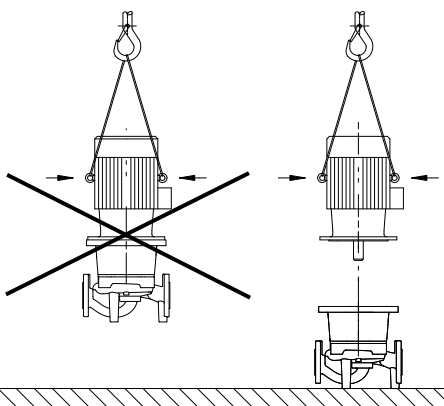
Fig. 2: Транспортировка электродвигателя
