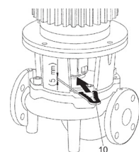
Asennushaarukka säätötöitä varten
