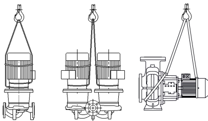
Fig. 1: Pumpun kuljetus
