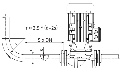
Fig. 9: Kevennysmatka ennen pumppua ja pumpun jälkeen
