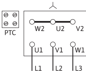
Fig. 11: Y-kytkentä
