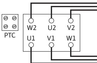
Fig. 12: Δ-liitântä
