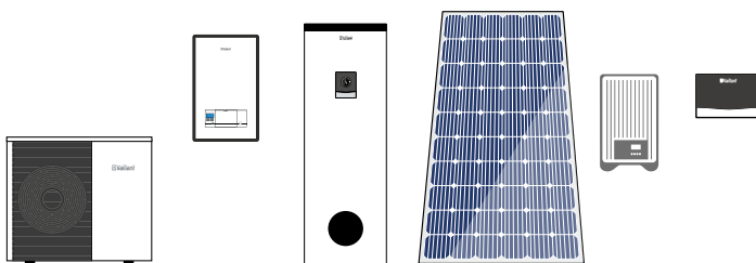
aroTHERM plus ze stacją hydrauliczną VVZ MEH 97, uniSTOR plus VIH RW, moduł fotowoltaiczny auroPOWER z falownikiem, sterownik systemowy sensoCOMFORT VRC 720
