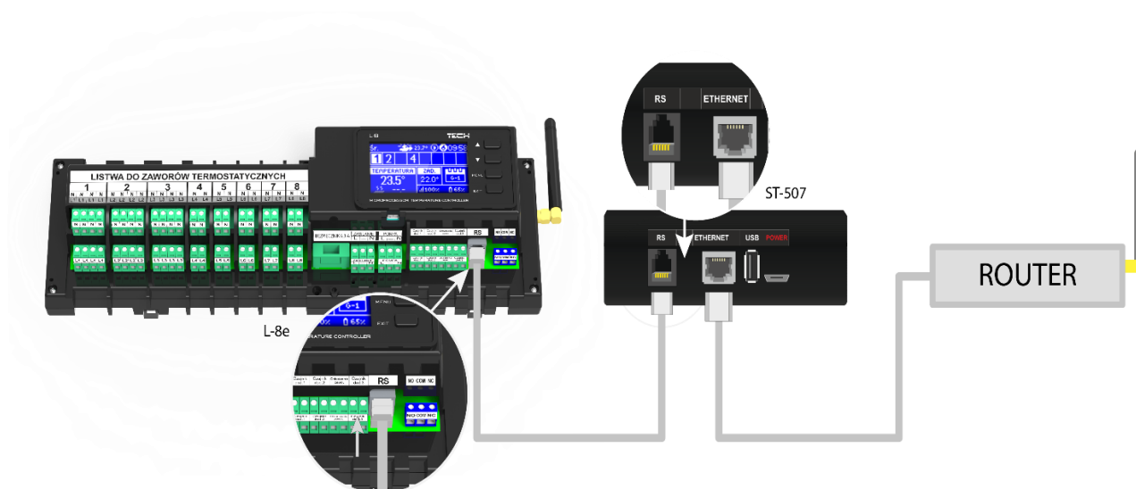
Schemat podpięcia modułu internetowego ST-507.
