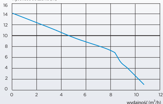
Ciśnienie wody wysokość tłoczenia (m)
