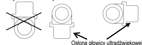
Rys. 6: Zalecana pozycja zabudowy w przypadku licznika zimna
