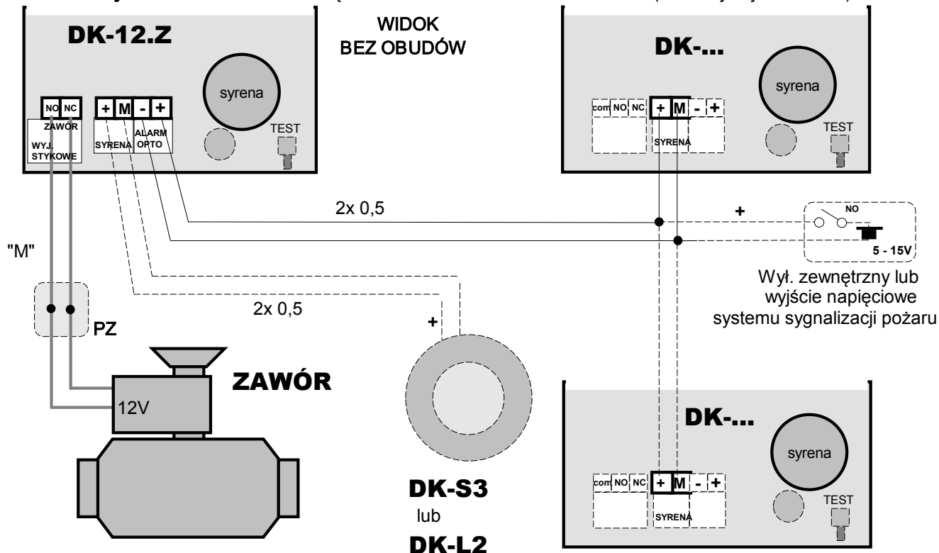
Rys 2.3.5 SCHEMAT POŁĄCZEŃ PRZEWODOWYCH DK- nn .Z (nie obejmuje zasilania):
