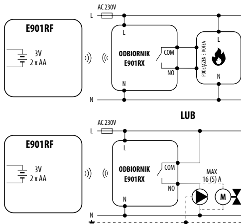
Schemat podłączenia dla regulatora bezprzewodowego E901RF
