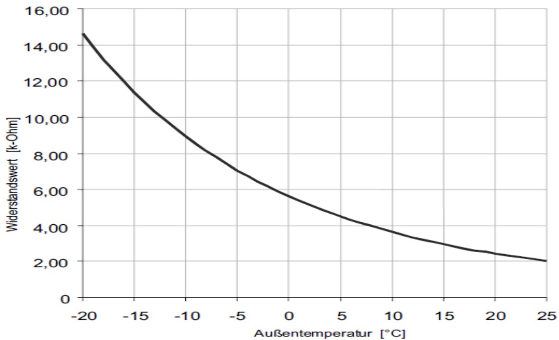
Abbildung: Fühlerkennlinie (DIN 44574) – Temperaturbereich -30°C – 35°C Drawing: Sensor characteristic (DIN 44574) – Temperature range -30°C – 35°C Figure: Caractéristique sonde (DIN 44574) - Gamme de température -30°C – 35°C
