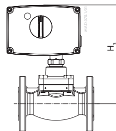
AMV 20/30 VB 2 (DN 15-50)
