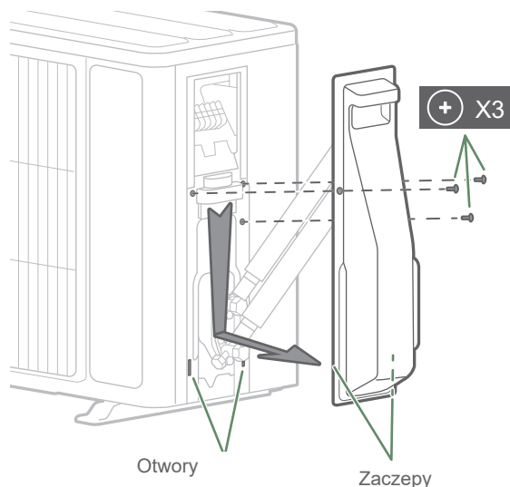
rys. 12 – Otwieranie jednostki zewnętrznej – modele 3, 5, 6 i 8
