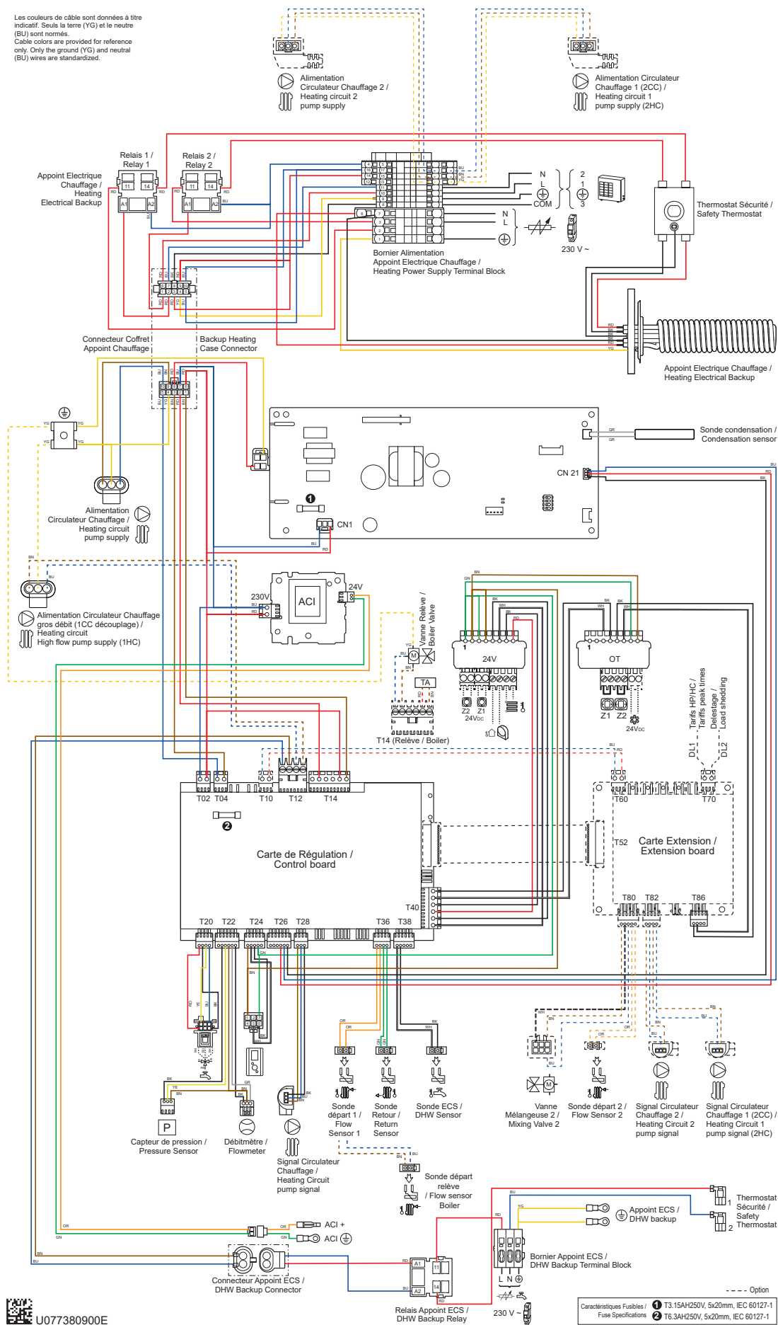
rys. 47 – Okablowanie elektryczne modułu hydraulicznego – Model jednofazowy
