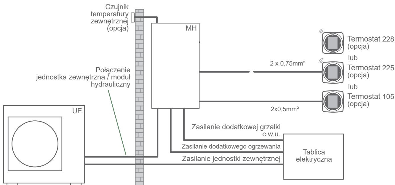
rys. 37 – Schemat połączeń elektrycznych dla prostej instalacji (1 obieg grzewczy)
