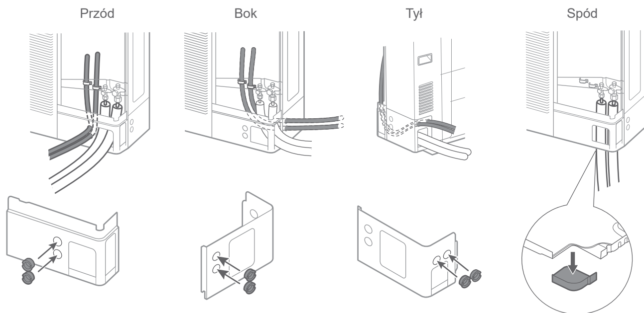
rys. 30 – Przejście połączeń chłodniczych jednostki zewnętrznej.
