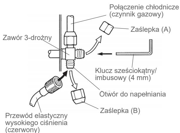
rys. 44 – Podłączenie przewodu elastycznego do zaworu czynnika gazowego
