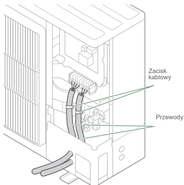
rys. 40 – Dostęp do listwy zaciskowej jednostki zewnętrznej
