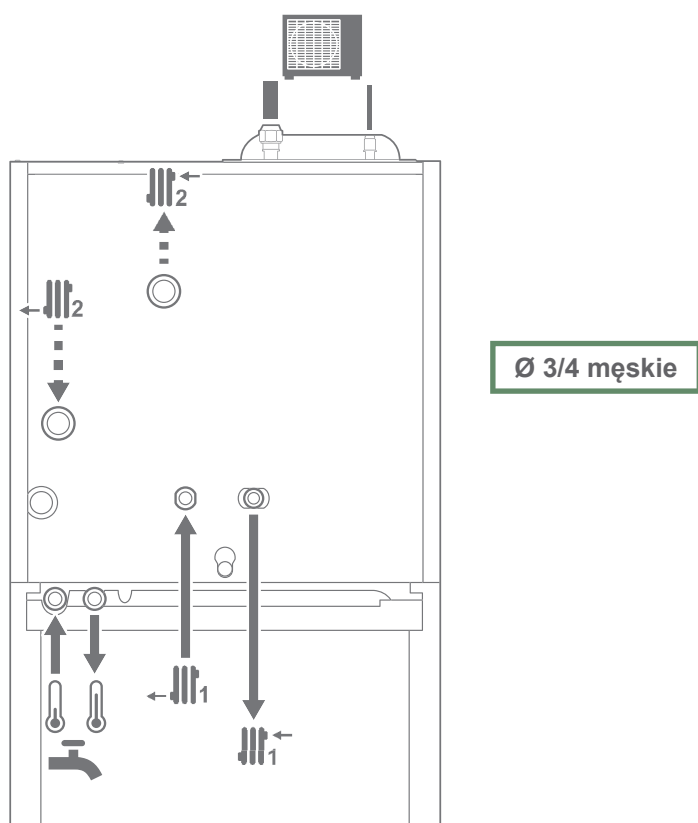
rys. 3 – Podłączenia hydrauliczne
