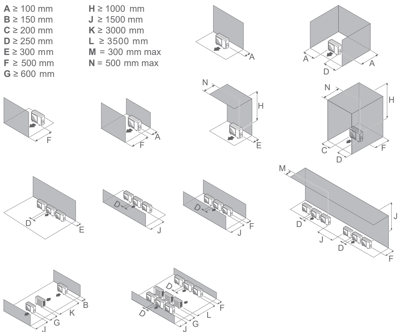
rys. 16 – Minimalne odstępy montażowe wokół jednostki zewnętrznej (model 10)
