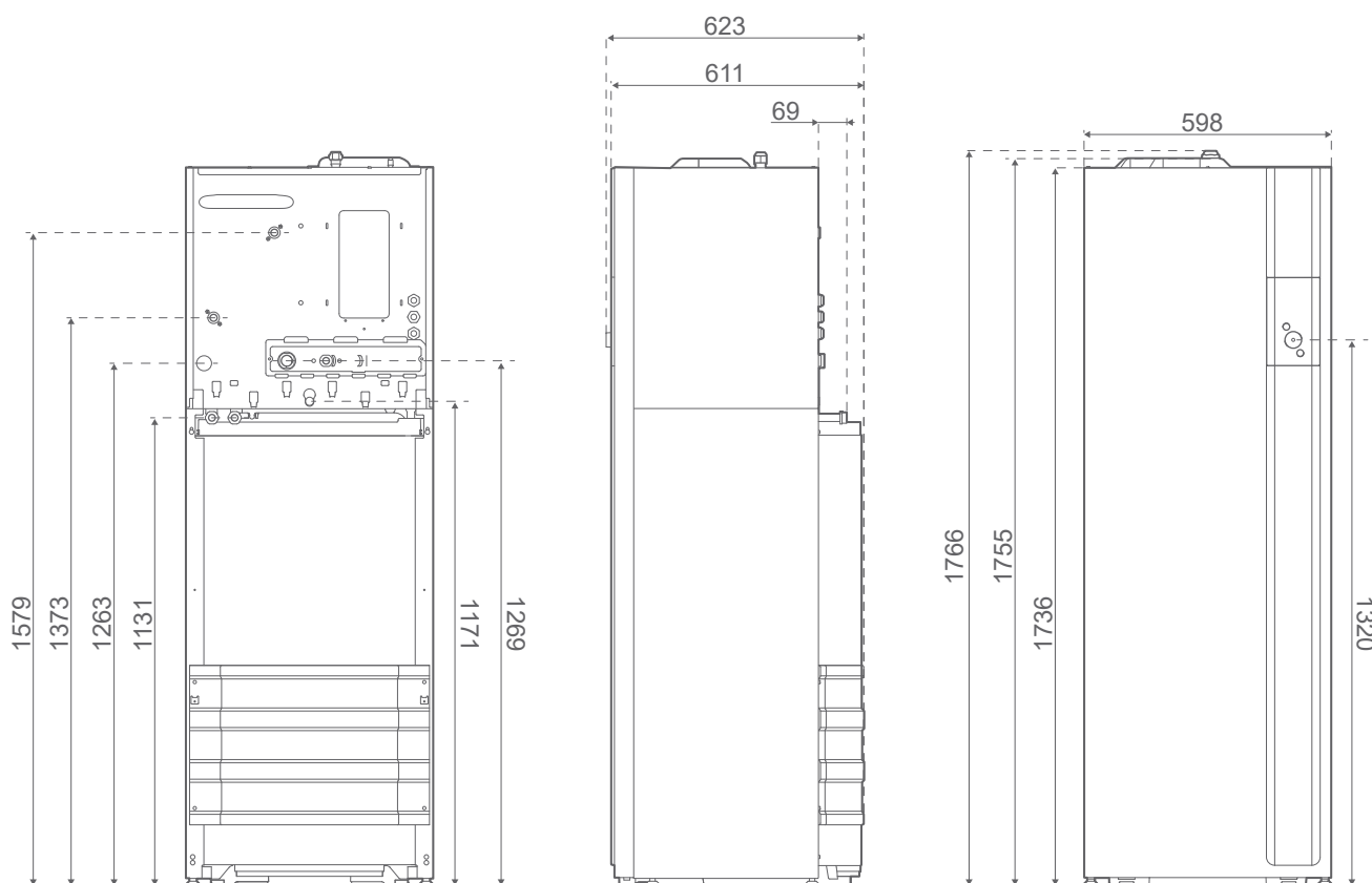
rys. 2 – Wymiary w mm
