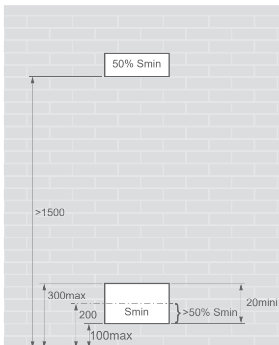
rys. 24 – Położenie otworów wentylacyjnych
