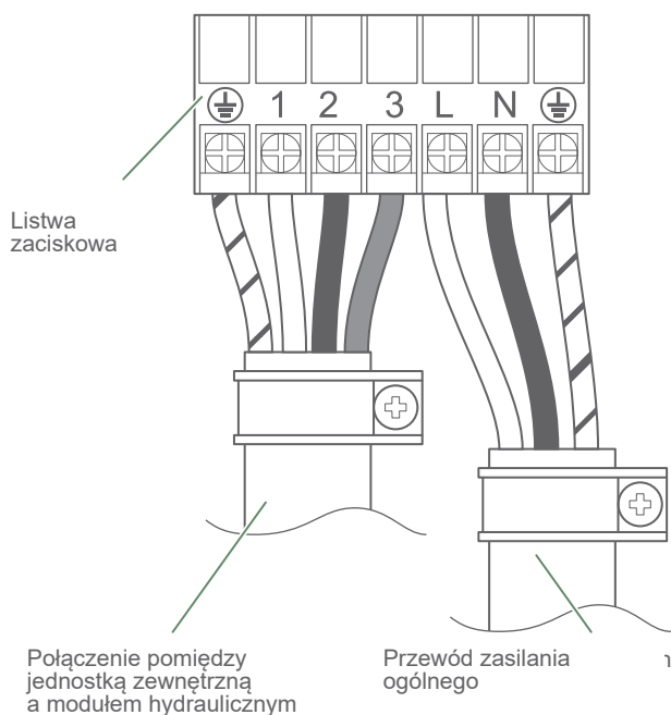
rys. 39 – Podłączenia do listwy zaciskowej jednostki zewnętrznej
