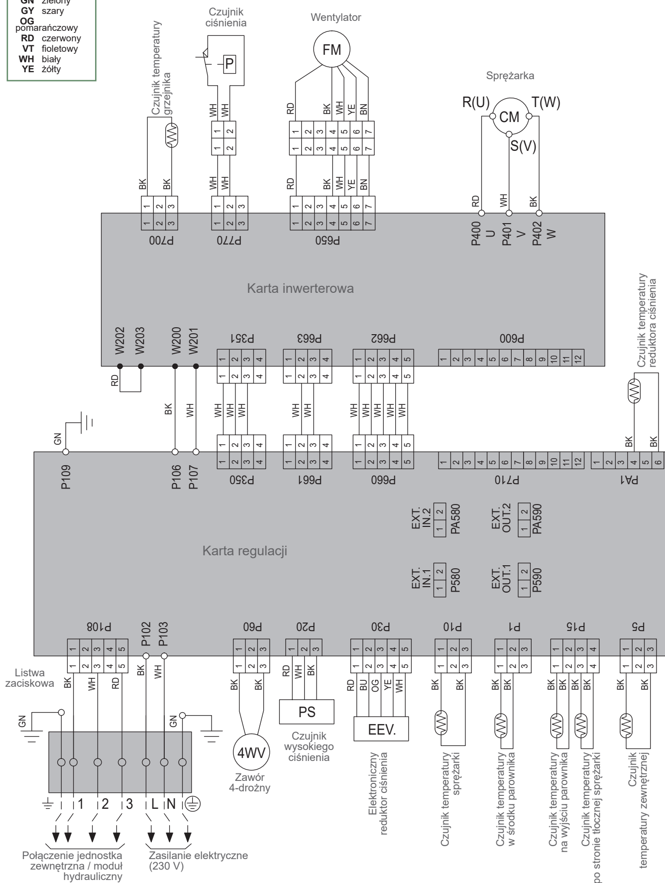
rys. 46 – Okablowanie elektryczne jednostki zewnętrznej – model 10
