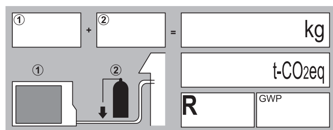
rys. 33 – Etykieta dodatkowej ilości czynnika chłodniczego
