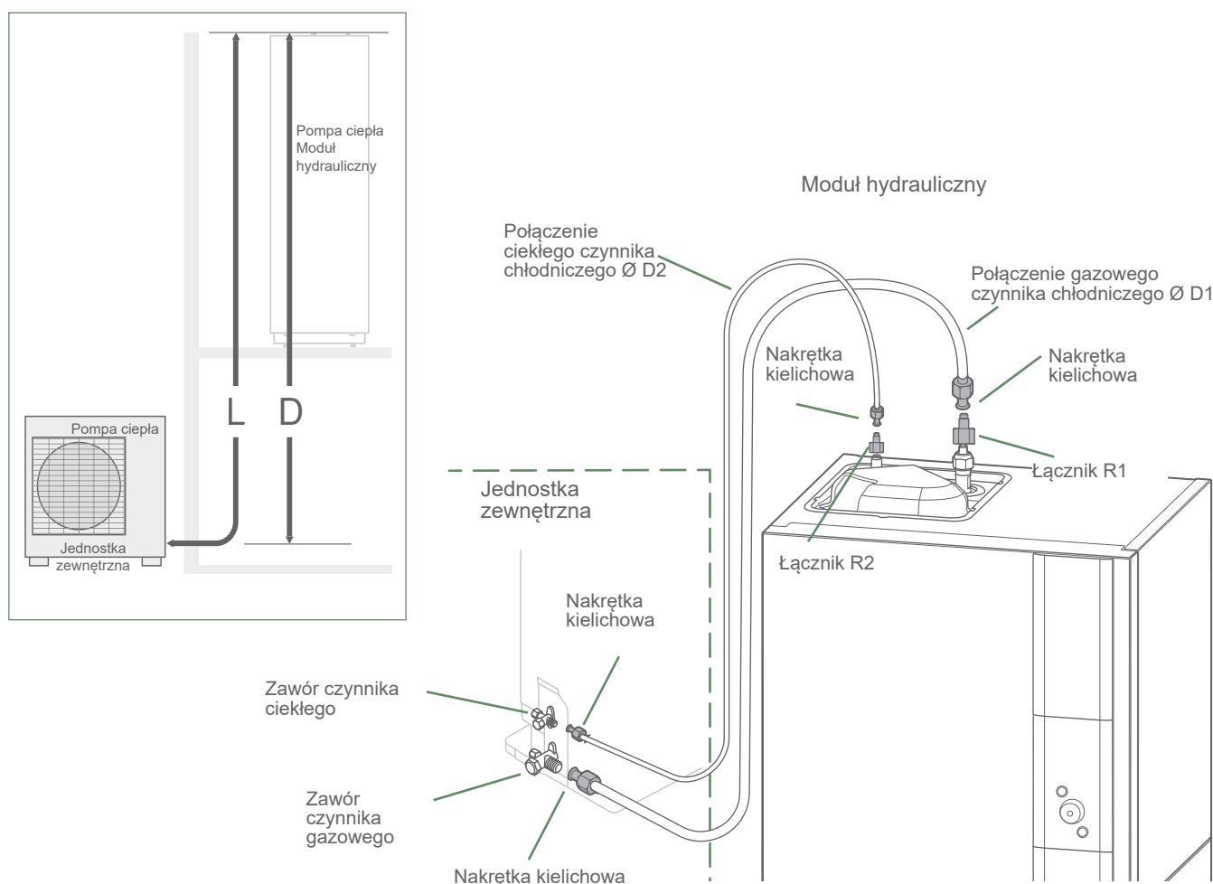
rys. 31 – Podłączenia połączeń chłodniczych (dopuszczalne średnice i długości)
